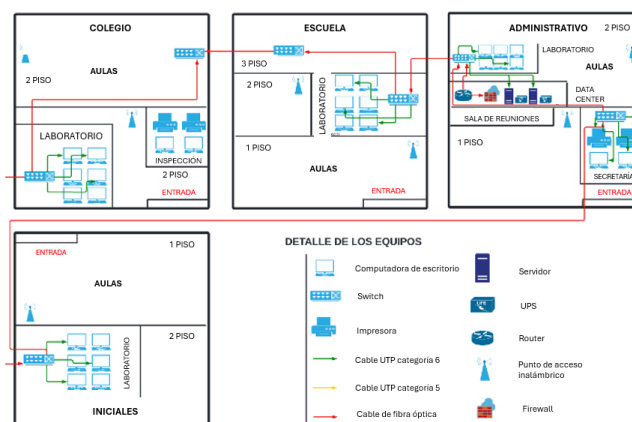
Figura 2. Diseño de red propuesto.
