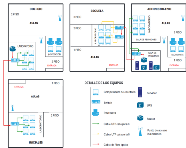
Figura 1. Infraestructura LAN actual
