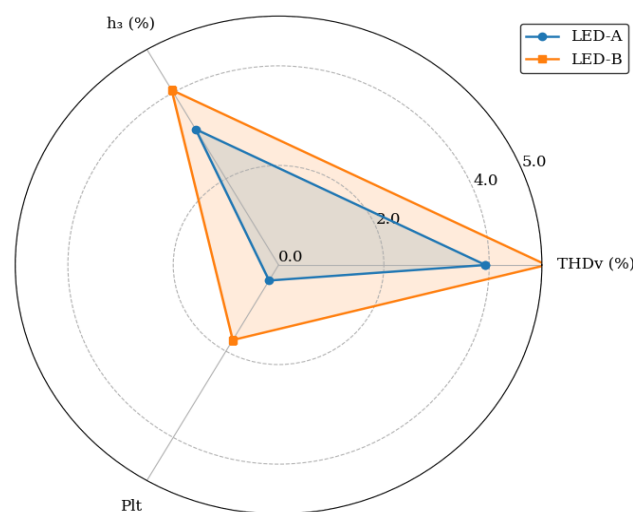
Figura 1. Comparación de parámetros eléctricos en operación continua.
