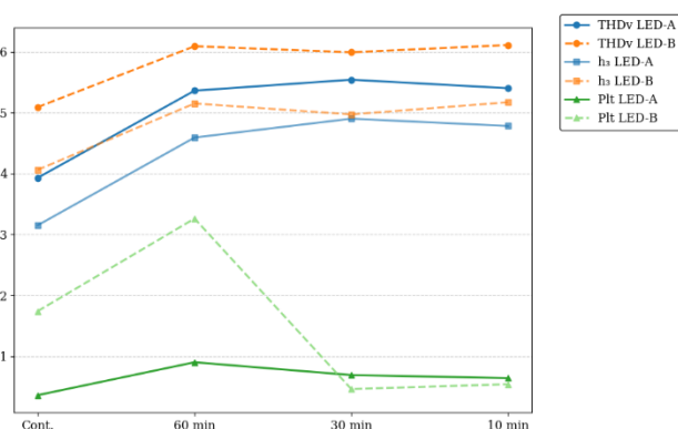
Figura 5. Evolución de parámetros eléctricos según régimen
