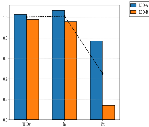
Figura 3. Relación normalizada 30/60 de parámetros eléctricos.
