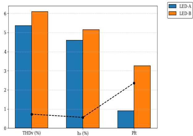
Figura 2. Comparación de parámetros en régimen de 60 min
