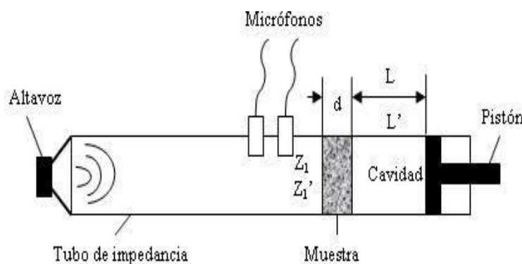
Figura 1. Esquema de disposición de tubo de medición acústica [9].
