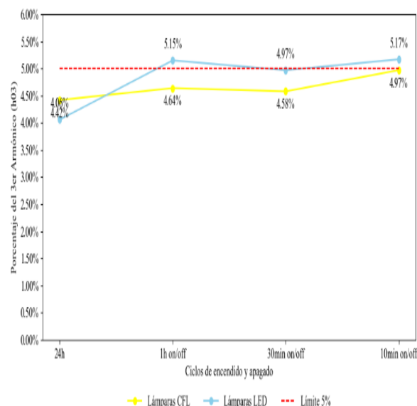
Figura 2. Comparación del componente armónico de tercer orden h3 según el ciclo y tipo de lámpara.
