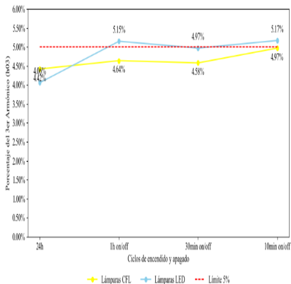
Figura 2. Comparación del componente armónico de tercer orden h3 según el ciclo y tipo de lámpara.
