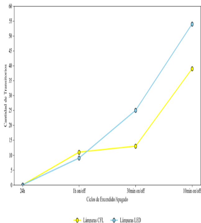
Figura 3. Variación del número de transitorios según el ciclo y tipo de lámpara.
