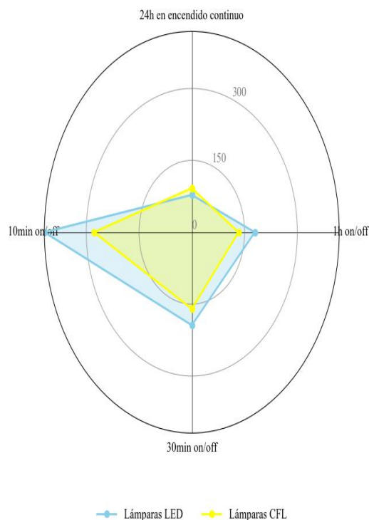
Figura 4. Comparación de la cantidad de eventos registrados por ciclo y tipo de lámpara.
